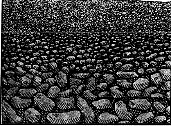
شكل (8): التطبق المتدرج
