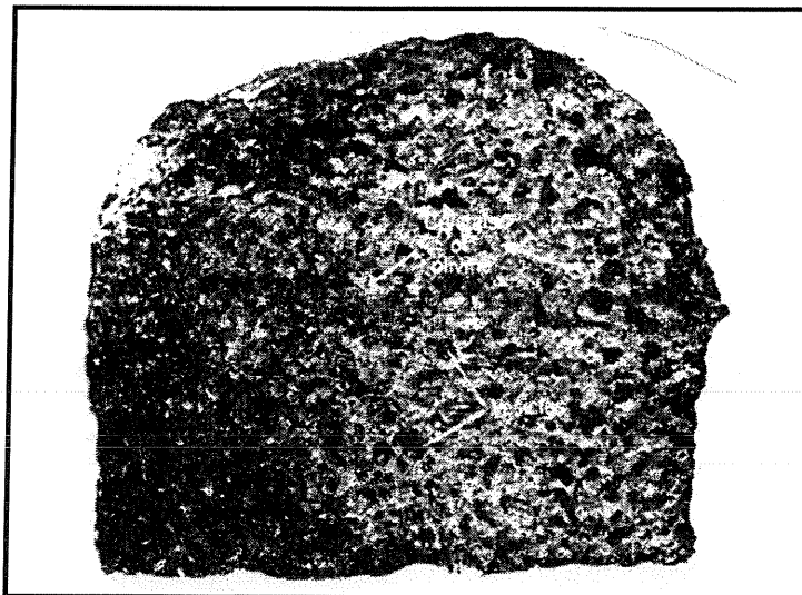
شكل (5): النسيج الفراغي في البازلت
