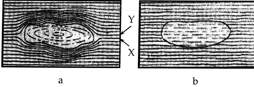
شكل (10): مقطع شاقولي يمر من جسمين تخثريين يظهر علاقتهما مع تطبيق الصخور الرسوبية
