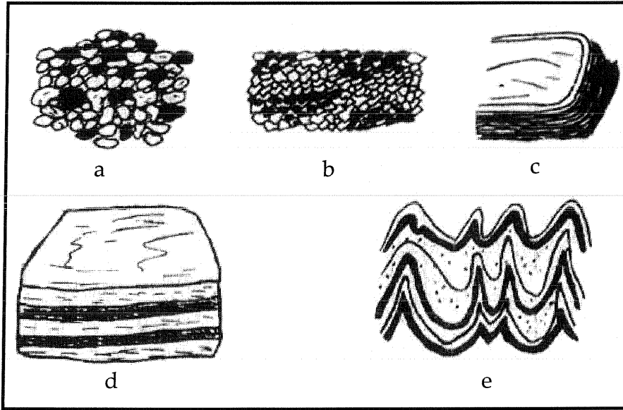
شكل (15): بعض أشكال النسيج في الصخور المتحولة
