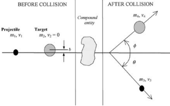
الشكل 1: التصادم بين قذيفة بكتلة m_1 وسرعة v_1 مع نواة هدف ساكنة v_2 = 0 بكتلة m_2 وتشكل وسيط يتفكك إلى جسيمان m_3 و m_4 ينطلقان بزاويتين \theta و \phi على الترتيب مع اتجاه القذيفة.
