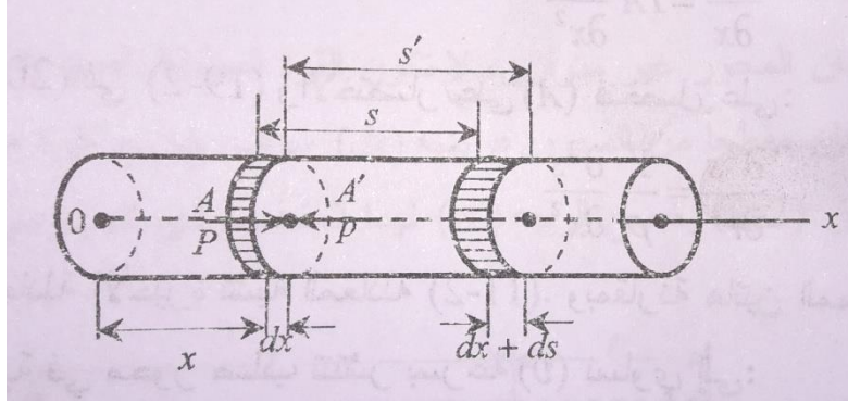
الشكل (3): أمواج الضغط في أسطوانة غاز.
