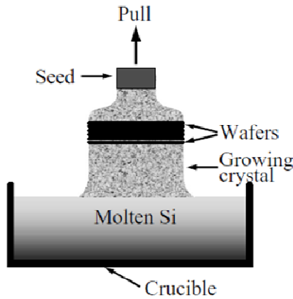
الشكل (1-5): طريقة تشوكرالسكي لإنماء أنصاف نواقل حجمية
