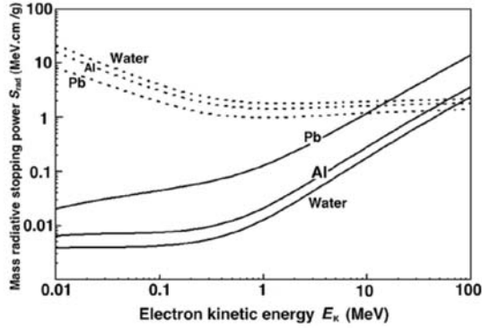
الشكل 2 قدرة التوقف الاشعاعية S_{rad} للالكترونات في أوساط الماء و الألمنيوم والرصاص بتابعة الطاقة الحركية للالكترون و هي ممثلة بخطوط مستمرة. تم رسم قوة التوقف التصادمية في نفس الأوساط للمقارنة و هي المنحنيات المرسومة بشكل نقطي.
