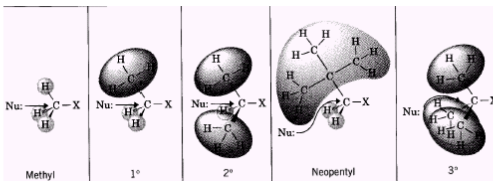
الشكل ( ٢ ) أثر بنية الركازة في تفاعلات \text{S}_\text{N}2
