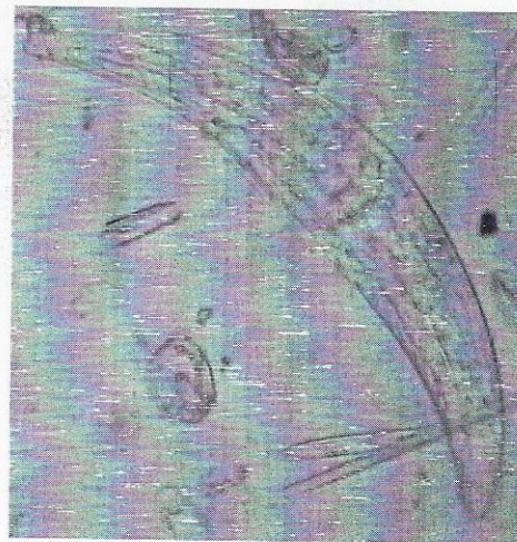
Closterium ehrenbergii
