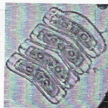
Achnanthes
