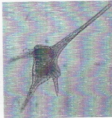
Ceratium
