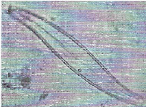
Cocconeis
