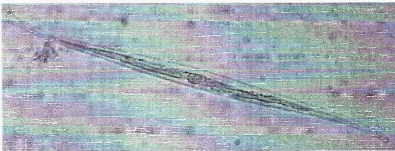
Nitzschia
