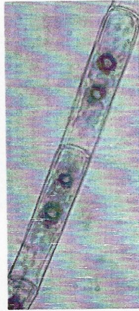
Zygnema
