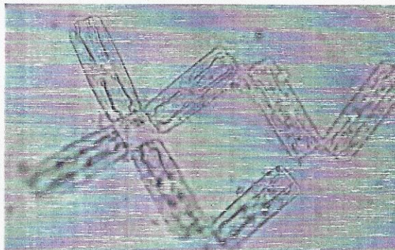
Frigilaria
