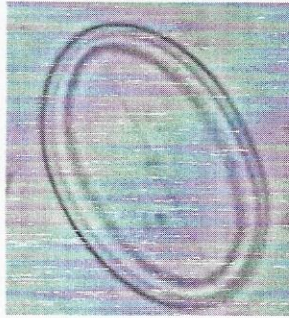
Cocconeis
