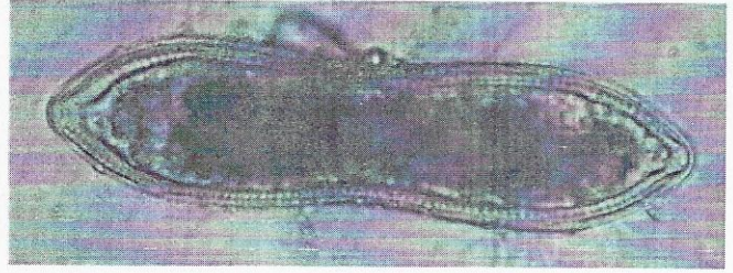
Cymatopleura
