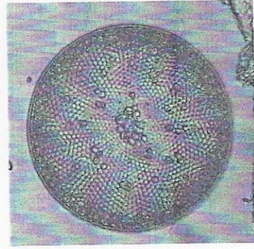
Thalassiosira
