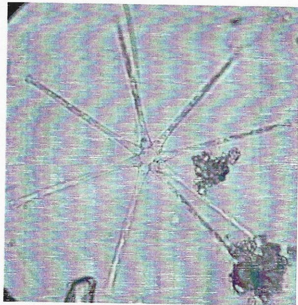
Asterionella
