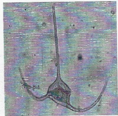
Ceratium
