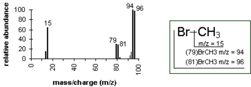
الشكل ( 7 - 28 ) الطيف الكتلي لبروم الميثان
