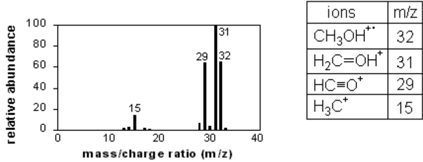
الشكل ( 7 - 27 ) الطيف الكتلي للميثانول
