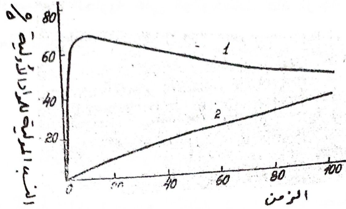
الشكل (4-1) الدراسة الحركية للتفاعل بين SiO_2, MgO
