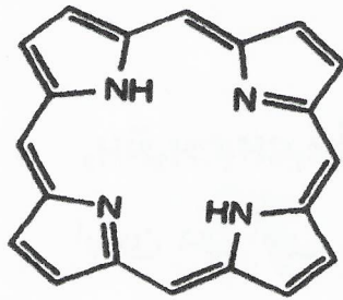
porphyrin
