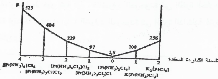
الشكل (١-١) العلاقة بين الناقلية الكهربائية وعدد الشوارد
