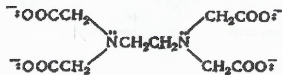
EDTA
