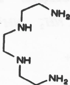
triethylenetetramine trien
